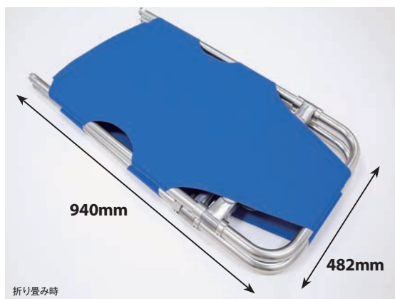
折り畳み時
